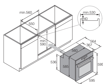
Installazione sottopiano
