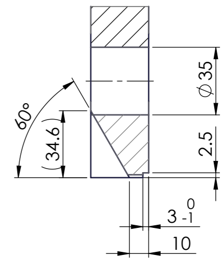
A-A (1 : 2)
