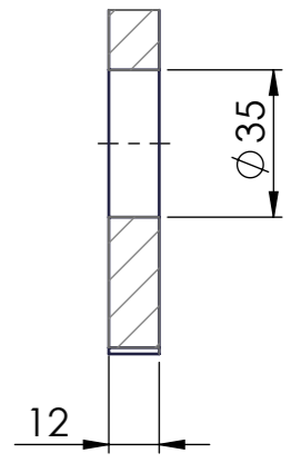
A-A (1 : 2)
