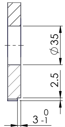
A-A (1 : 2)
