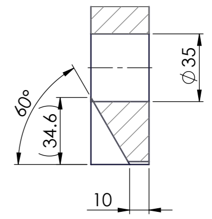
A-A (1 : 2)
