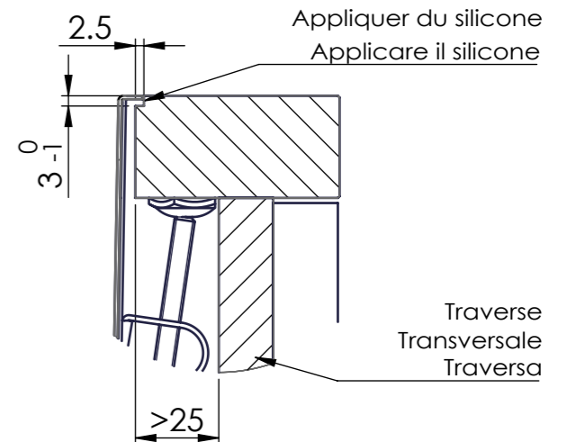
Y (1:2)
